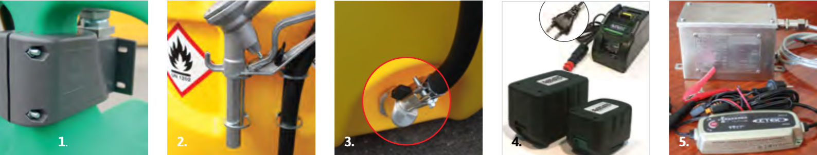
1. Кронштейн для ручного и электронасоса. Manual and electric pump holder. 2. Держатель для пистолета. Nozzle holder. 3. Шаровый кран безопасности. Safety ball valve with turning joint. 4. Перезарядные батареи на 12 или 24 В для заправки до 550 или 1100 л. Зарядное устройство (12-24 В) от прикуривателя автомобиля или с вилкой 220 В. Rechargeable batteries at 12 or 24 V, for deliveries up to 550 or 1100 litres and battery charger (12-24 V) with car lighter socket or standard 220 V plug. 5. Бензиновое исполнение: в наличии с питанием от аккумулятора с сертификацией АТЕХ, 12 В, с подзарядкой. Gasoline version: available with power supply by rechargeable battery, ATEX certified, 12 V. 6. Крышка заливной горловины со встроенным вентиляционным клапаном. Filling plug with integrated vent device. 7. Верхняя ручка для удобства захвата и подъема. Top handle for easy gripping and lifting.
